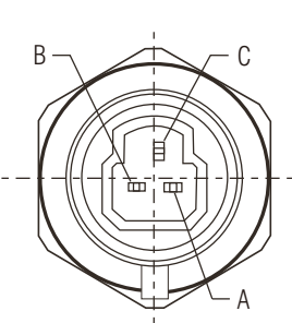
Packard接头 插头型号:DELPHI 120078088
