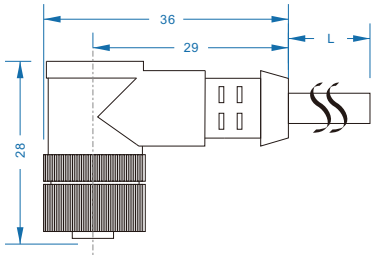
直角型带线
