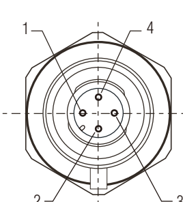
M12-4P温压一体航空插座
