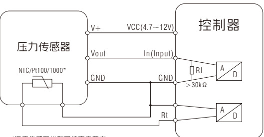
温压一体接线
